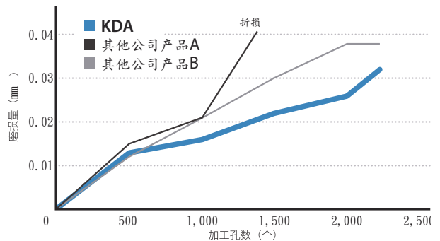
耐磨損性对比 (本公司对比)
